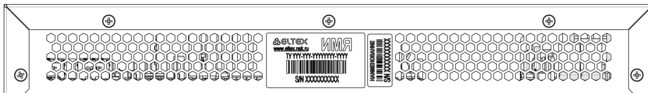
Рисунок 25 – Задняя панель MES2408, MES2408B, MES2408C, MES2408CP, MES2408PL
