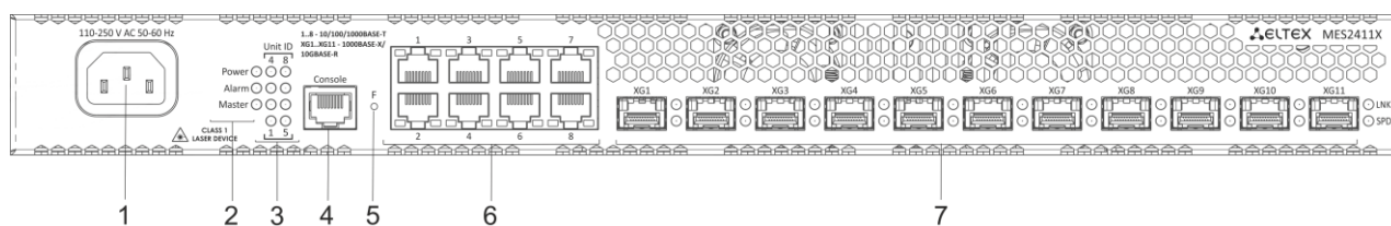
Рисунок 23 – Передняя панель MES2411X
