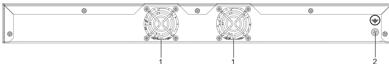
Рисунок 26 – Задняя панель MES2424P, MES2428P
