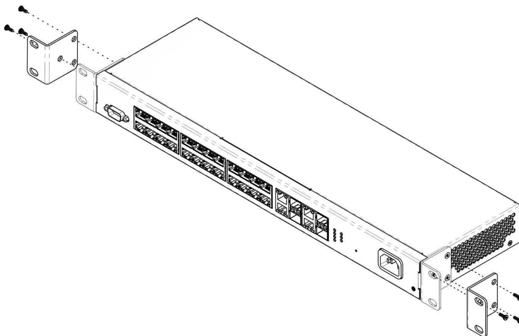
Рисунок 36 – Крепление кронштейнов
