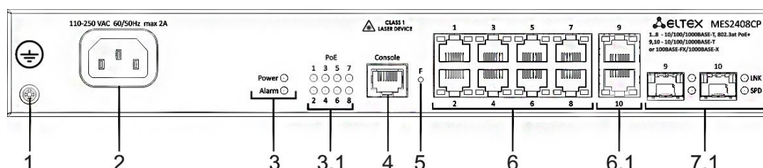
Рисунок 6 – Передняя панель MES2408CP
