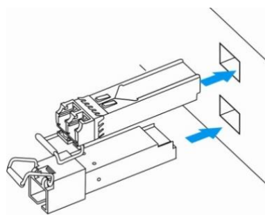
Рисунок 39 – Установка SFP-трансиверов
