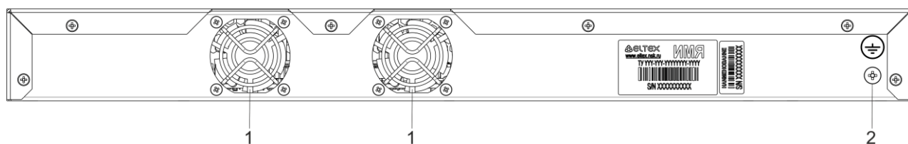
Рисунок 30 – Задняя панель MES2411X
