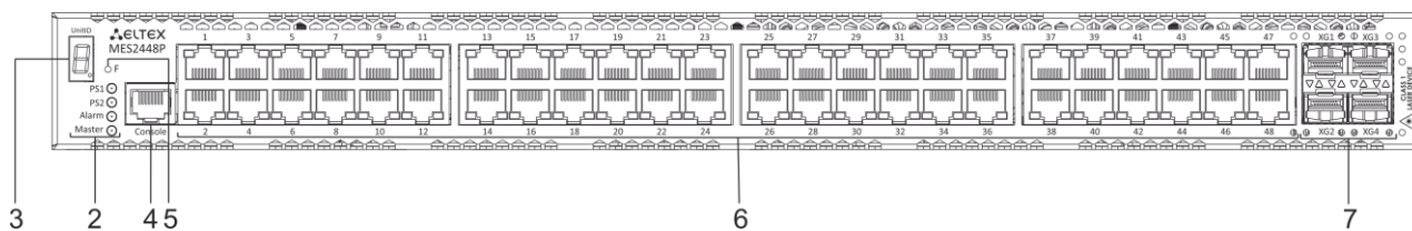
Рисунок 22 – Передняя панель MES2448P
