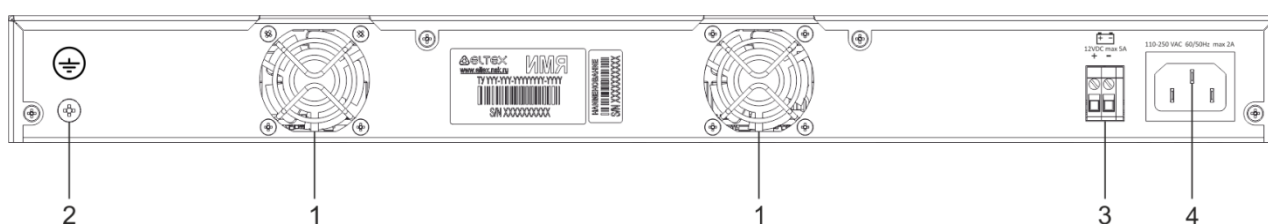
Рисунок 28 – Задняя панель MES2448B
