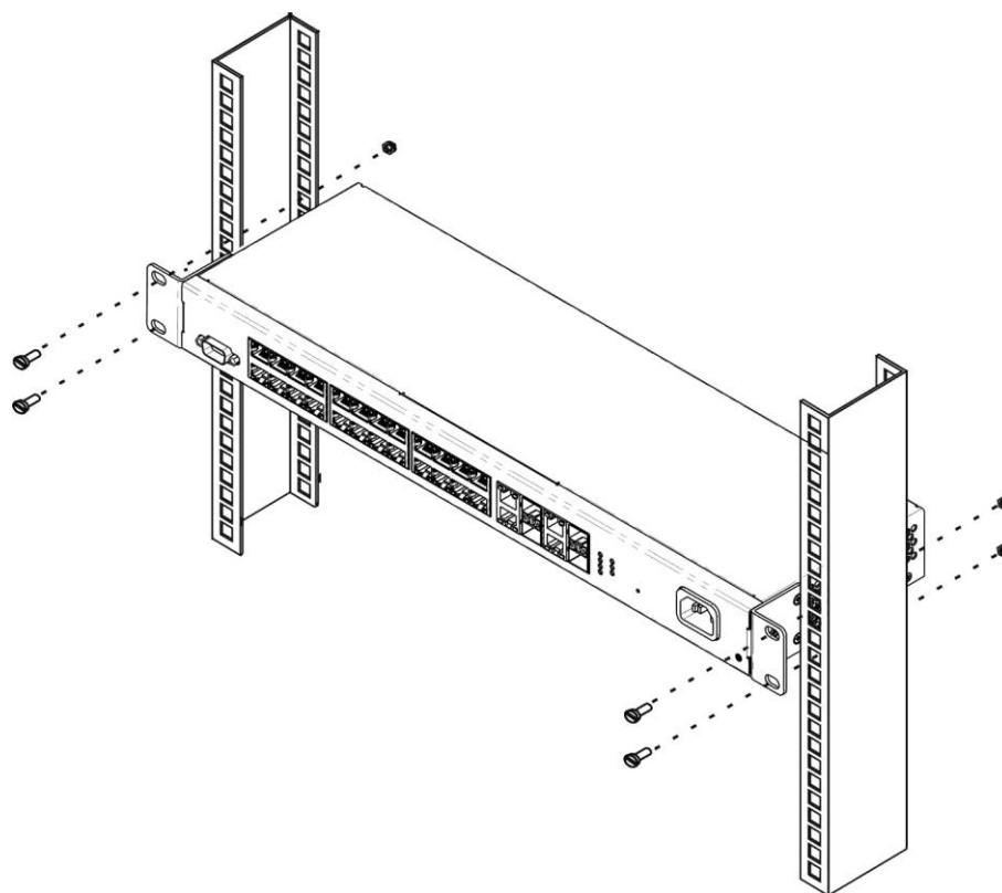
Рисунок 37 – Установка устройства в стойку
