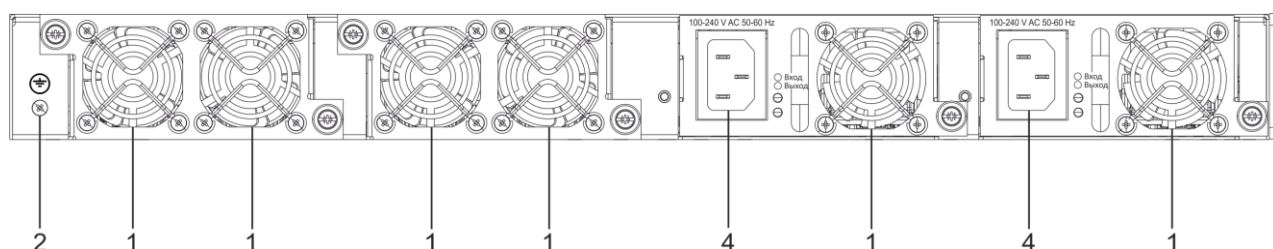
Рисунок 29 – Задняя панель MES2448P
