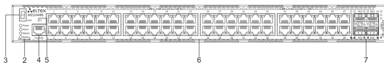
Рисунок 21 – Передняя панель MES2448B
