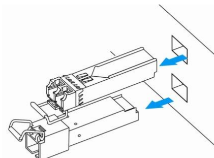
Рисунок 42 – Извлечение SFP-трансиверов
