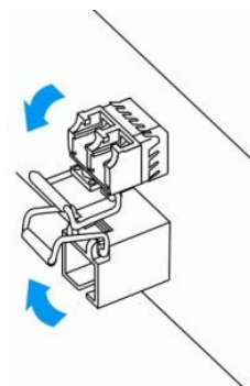
Рисунок 41 – Открытие защелки SFP-трансиверов
