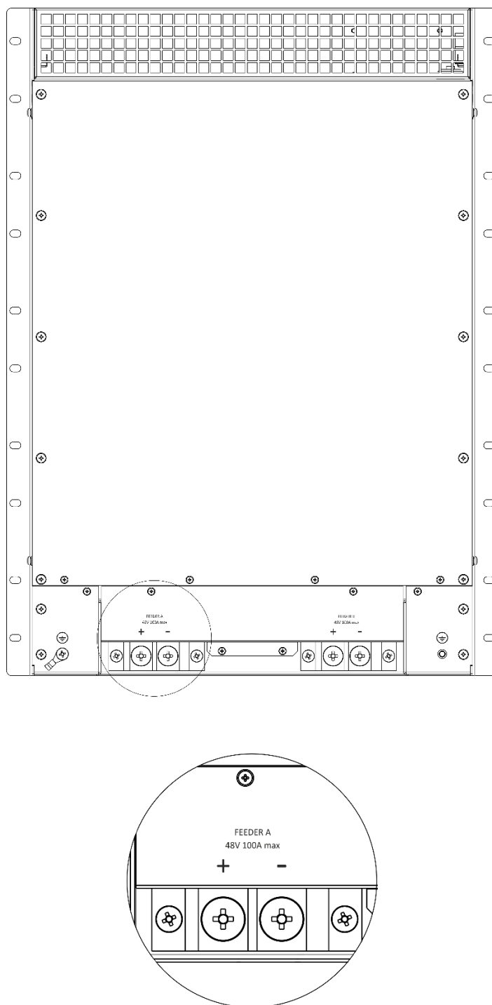
Рисунок 27 — Подключение ME5000, ME5000M к питающей сети
