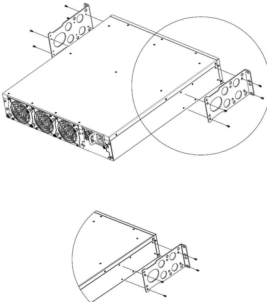
Рисунок 21 — Крепление кронштейнов
