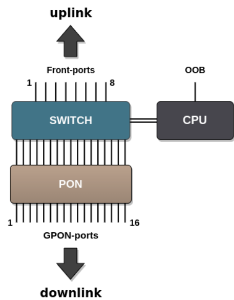
Рисунок 24 – Набор интерфейсов терминала
