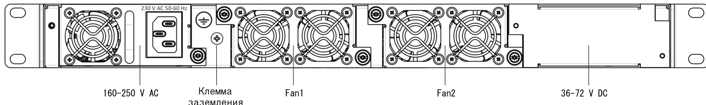
Рисунок 11 – Задняя панель терминала LTX-8(16)
