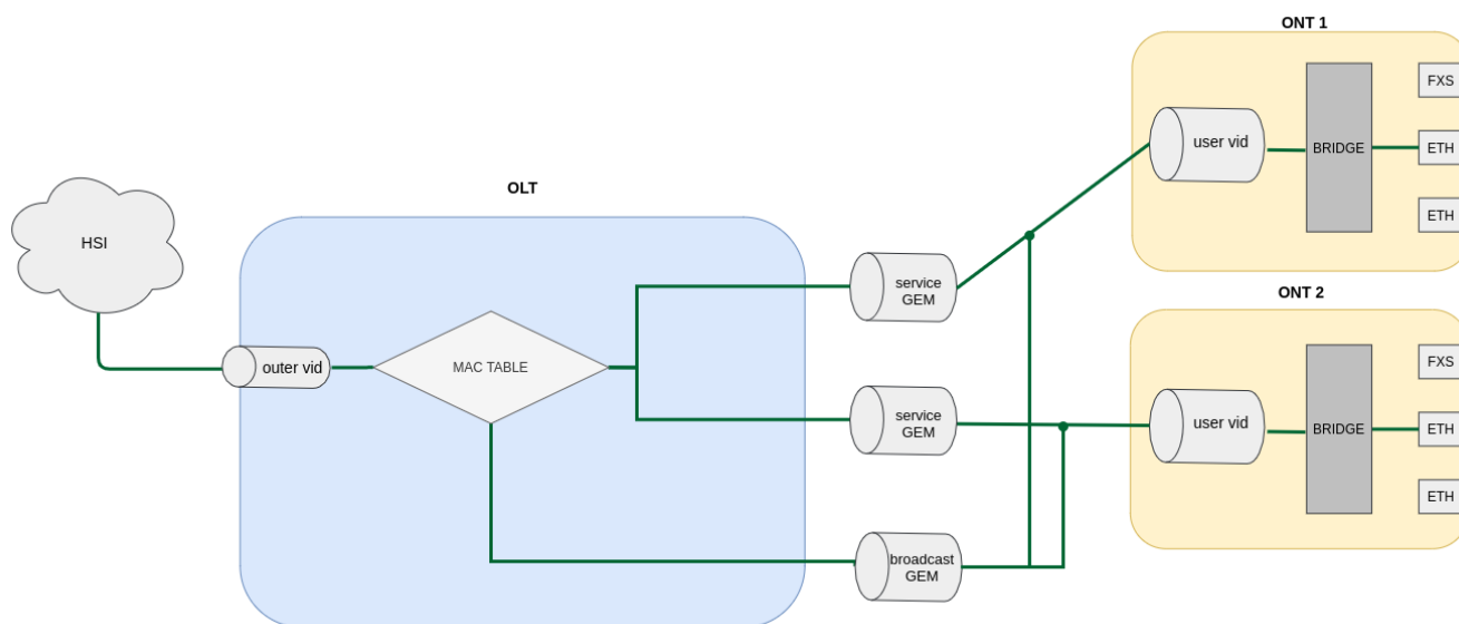
Рисунок 27 – Схема модели N-to-1
