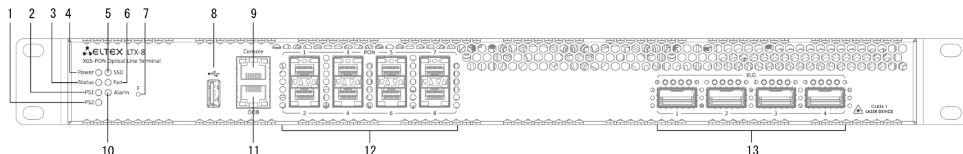
Рисунок 10 – Передняя панель терминала LTX-8
