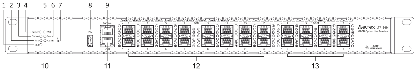
Рисунок 1 – Передняя панель терминала LTP-16N
