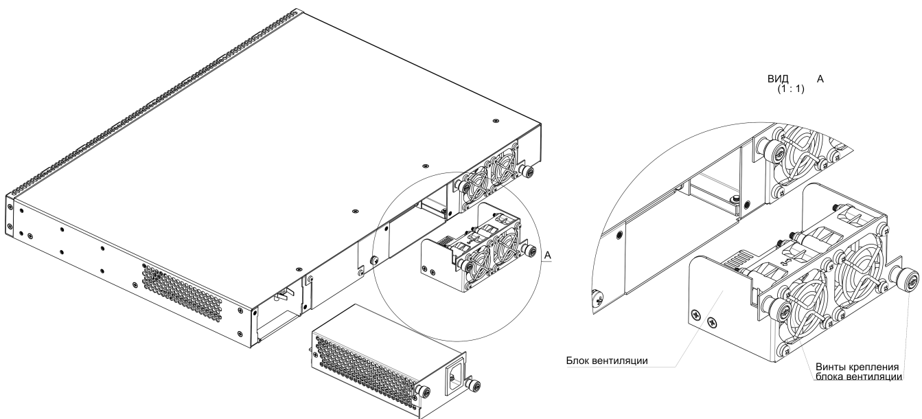
Рисунок 34 – Блок вентиляции. Крепление в корпус
