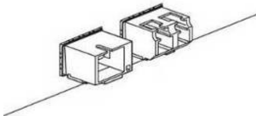
Рисунок 31 – Установка SFP-трансиверов
