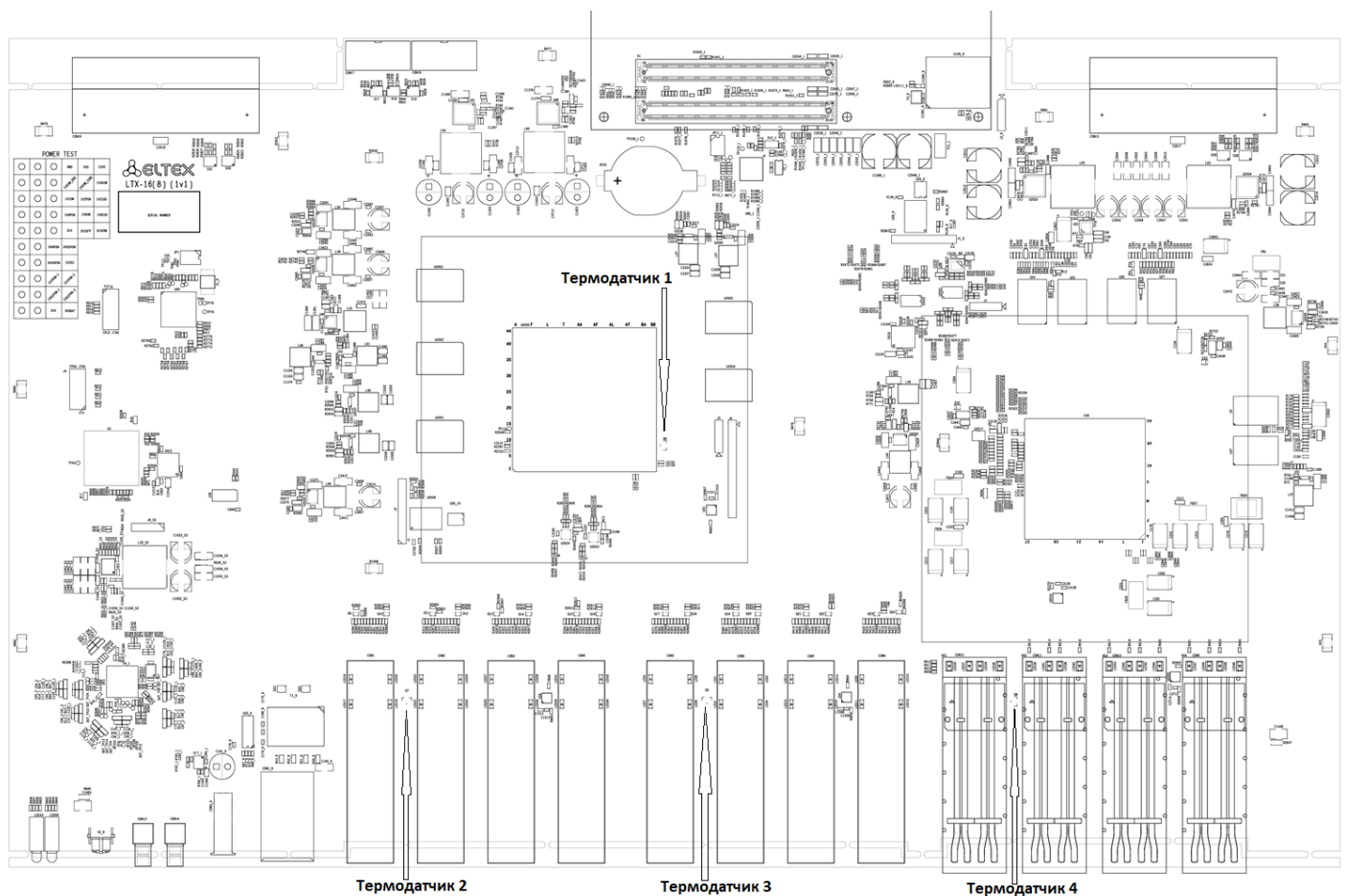
Рисунок 12 – Расположение термодатчиков LTX-8(16)
