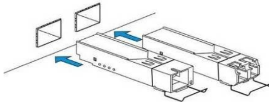
Рисунок 30 – Установка SFP-трансиверов
