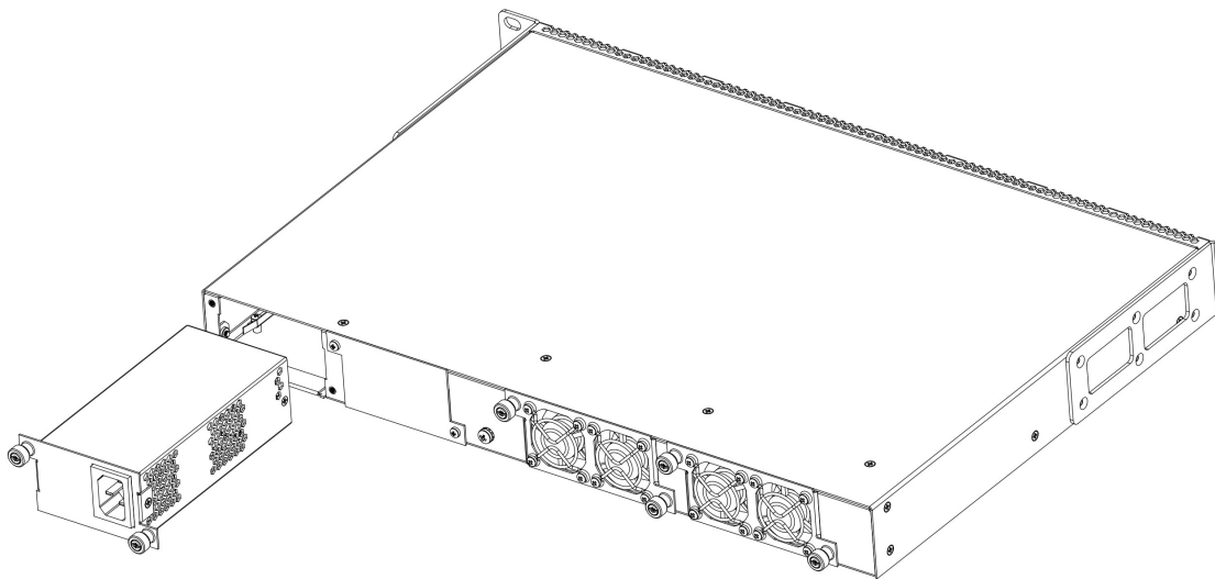
Рисунок 6 – Установка модуля питания в LTP-16N(T)
